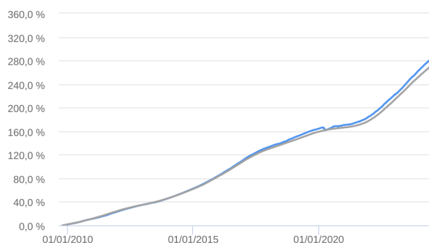
Retorno Acumulado - 15/10/2009 a 28/06/2024 (diária)
